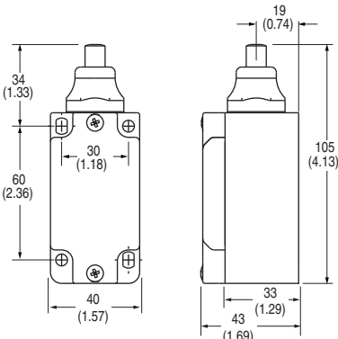
Dome Plunger
