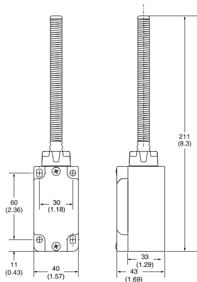
Spring Rod
