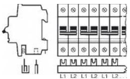
SZ-PSB 53 N, SZ-PSB 54 N SK 0098 Z96 SZ-PSB 55 N, SZ-PSB 56 N 1-pole + NA or 2-pole with 2 phases or 1 phase + N
