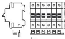
SZ-KS 18/12 N SK 0202 Z99 SZ-KS 18/56 N 1-pole with 1 phase
