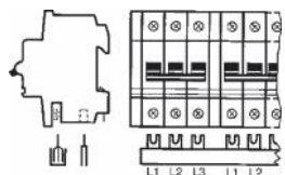
SZ-PSB 49 N, SZ-PSB 50 N SK 0097 Z 96 SZ-PSB 51 N, SZ-PSB 52 N 3-pole + aux.sw.. with 3 phases
