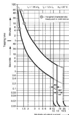
S 220-K 10 ... 16 A
