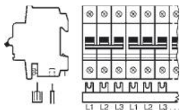
SZ-PSB 3 N, SZ-PSB 4 N SK 0139 Z96 SZ-PSB 11 N, SZ-PSB 12 N 1- or 3-pole with 3 phases
