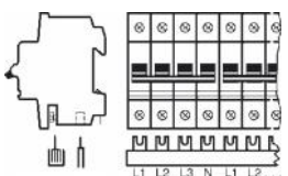
SZ-PSB 61 N, SZ-PSB 62 N SK 0101 Z96 SZ-PSB 63 N, SZ-PSB 64 N 3-pole + NA or 4-pole with 4 phases or 3 phase + N
