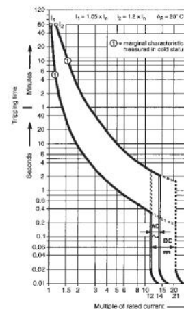
S 220-K 20 ... 32 A
