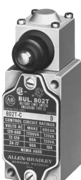
Side Push Rod
