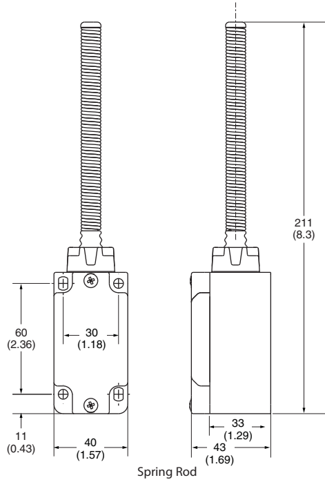
Spring Rod
