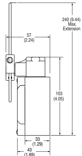
Rod Lever
