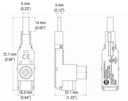
1489-AMCLT35
