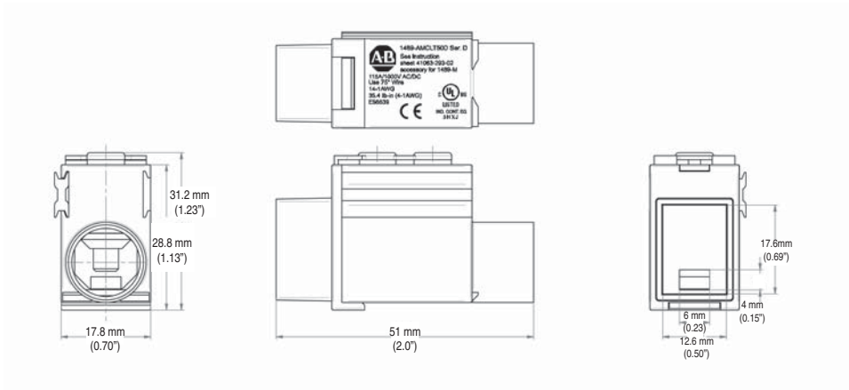
1489-AMCLT50D
