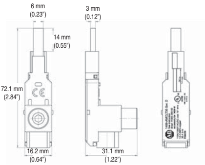
1489-AMCLT35
