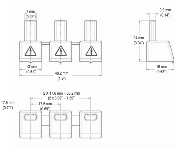
1489-AMCLPS
