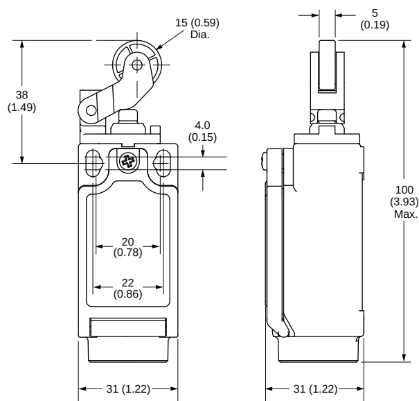
Hinge Lever
